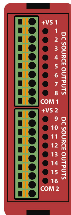
EZRPL-IO-16DCOP
