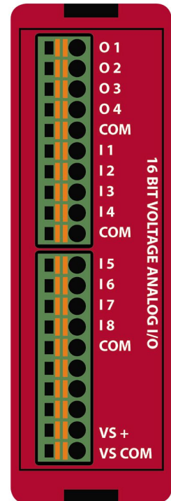
EZRPL-IO-8ANI4ANOV-16BIT
