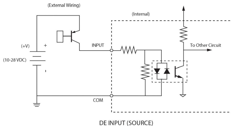
EZRPL-IO-16DCI
