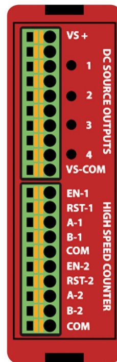
EZRPL-IO-HSCNT
