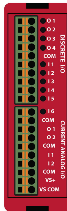
EZRPL-IO-6DI4DO-2ANI2ANOC
