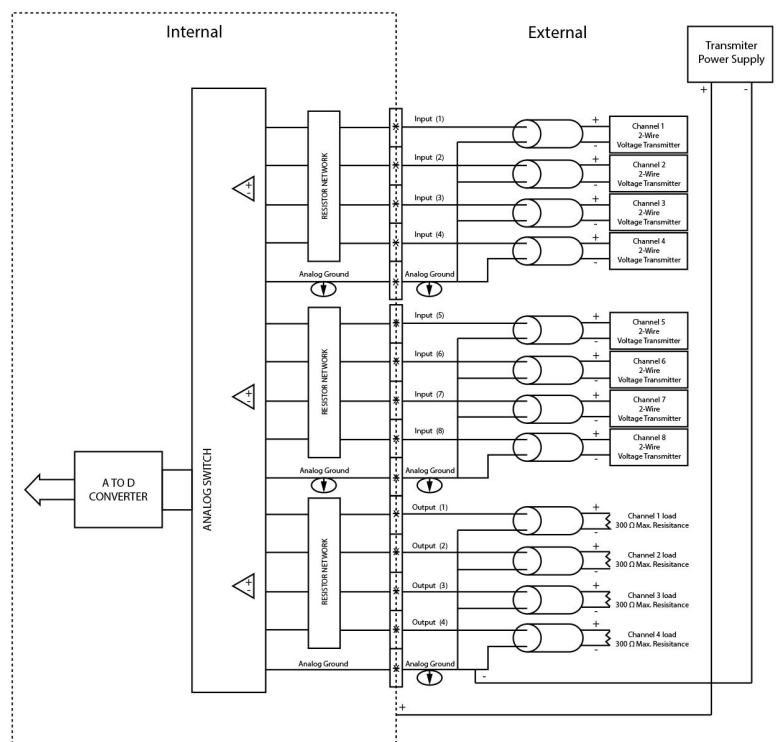
EZRPL-IO-8ANI4ANOV-16BIT
