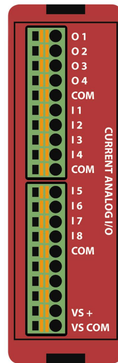
EZRPL-IO-8ANI4ANOC-16BIT
