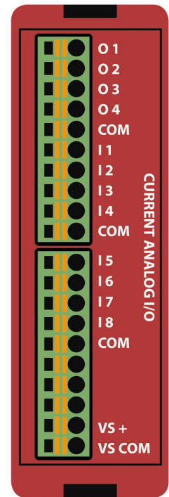
EZ RPL-IO-8ANI4ANOC
