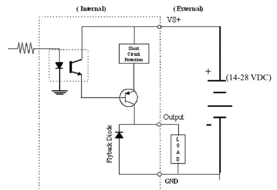
Output Wiring
