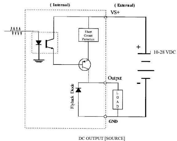
EZRPL-IO-4DCOP4RLO
