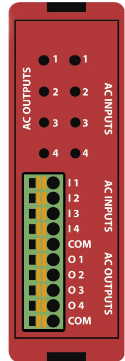
EZRPL-IO-4ACI4ACO
