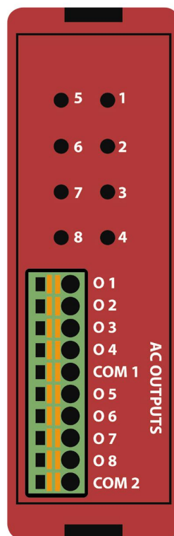
EZRPL-IO-8ACO
