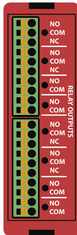
EZRPL-IO-8RLO
