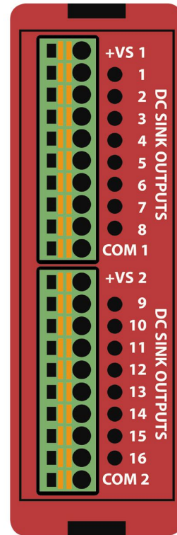
EZRPL-IO-16DCON
