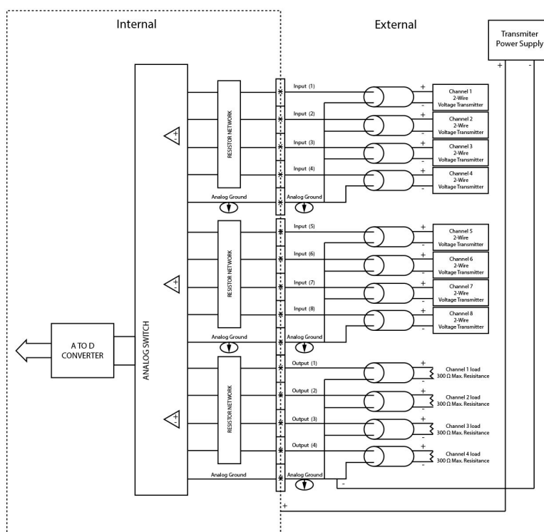
EZRPL-IO-8ANI4ANOV
